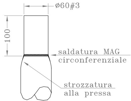
Particolare lavorazione cima palo
