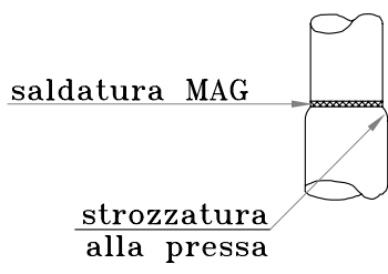
Particolare rastremature R
