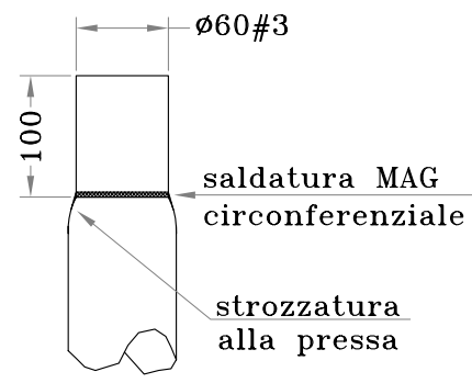
Particolare lavorazione cima palo
