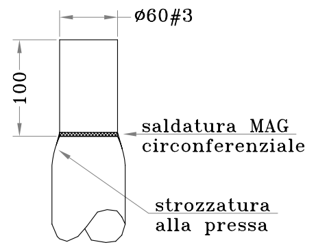
Particolare lavorazione cima palo
